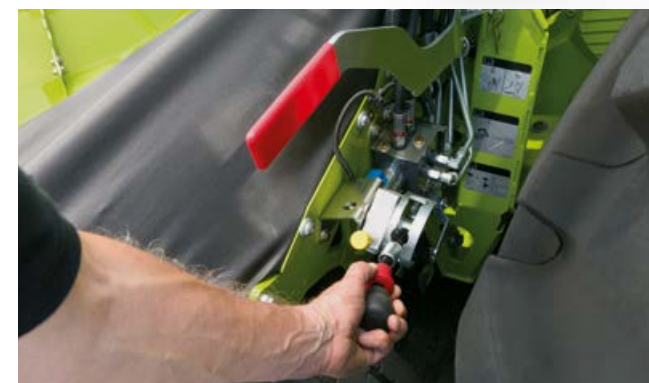
喂入塔轮转速三级可调，实现最佳作物流。
